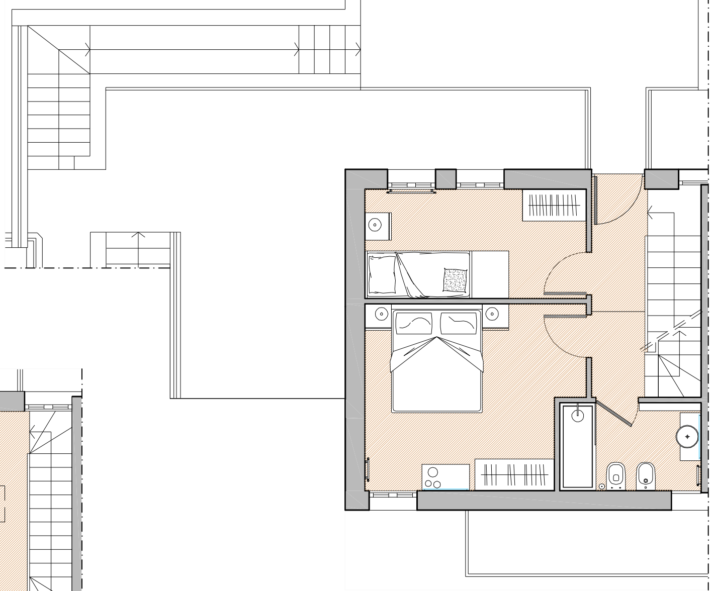
PIANO PRIMO
